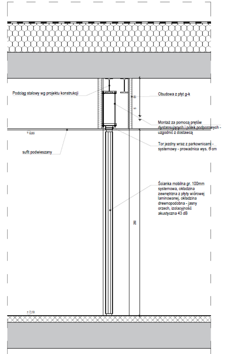
DETAL MOCOWANIA ŚCIANKI MOBILNEJ - 1:20
